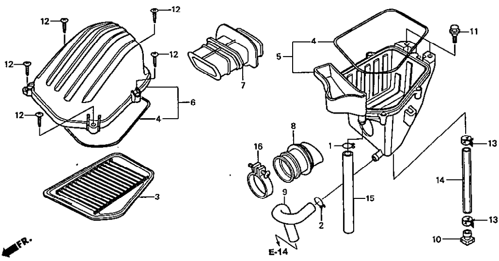
F - 17 ไส้กรองอากาศ Air Cleaner
